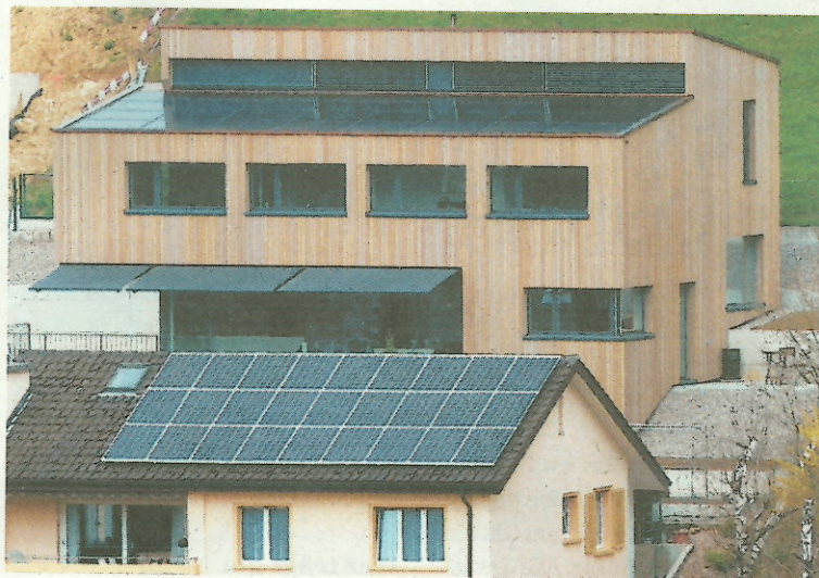
Neubau (hinten) – Indach-PV-Anlage, vorne Aufdach-PV-Anlage.
